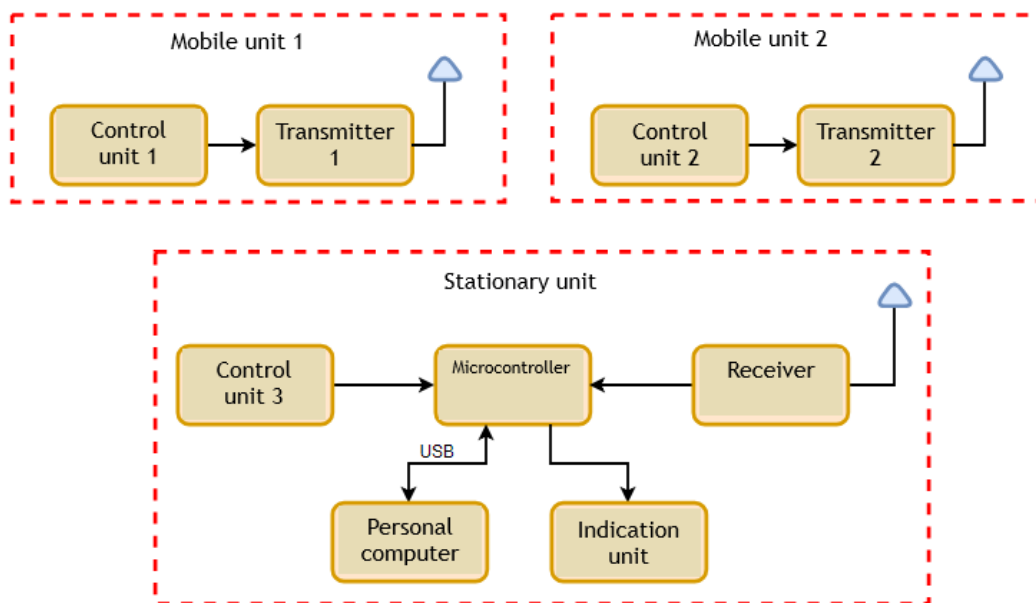
Рис 3. Структурна схема пристрою
