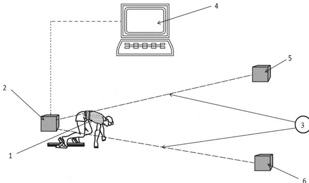
Рис. 2. Структурна схема конструктивного рішення пристрою для контролю спеціальної швидкісної витривалості:
